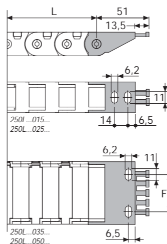
Fig. A Fissaggio della catena sull'esterno raggio. (Fig A) Vedi varianti di montaggio a pag. 31.
